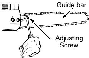
Guide bar
